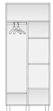
Cod. ADRF332 Armadio a 1 anta e 5 ripiani L900 x P560 x H2326 mm
