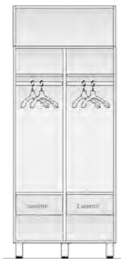
Cod. ADR322 Armadio a 2 ante e 2 cas. L900 x P560 x H2326 mm
