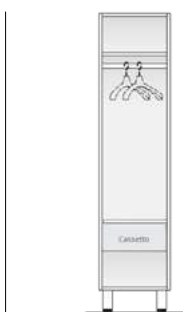
Cod. ADRA12 Armadio a 1 anta e 1 cas. L450 x P560 x H1910 mm
