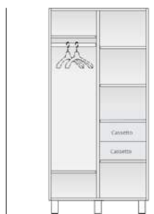
Cod. ADRF35 Arm. a 2 ante, 2 cas. e 5 rip. L900 x P560 x H1910 mm
