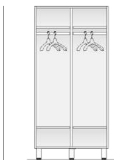
Cod. ADRF20 Armadio a 2 ante L900 x P560 x H1910 mm
