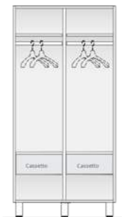
Cod. ADR622 Armadio a 2 ante e 2 cas. L900 x P560 x H1910 mm
